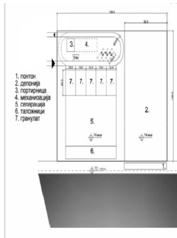
Слика 2: Шематски приказ депоније речног материјала □ типа Б
